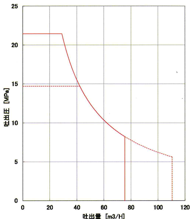
●ポンプ能力線図
